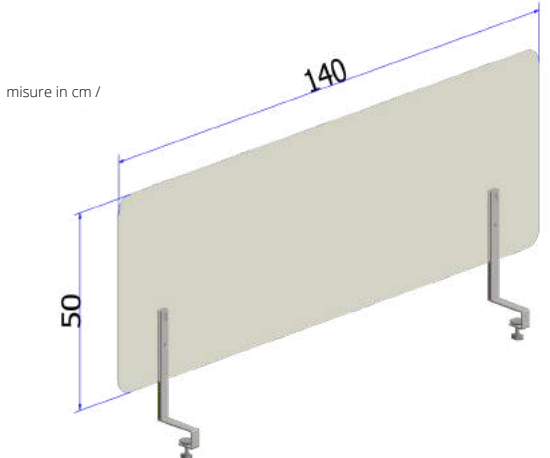
pannello con morsetti da aggancio sospeso dal top per facilitare il passaggio dei documenti / Panel with clamps suspended from top to facilitate document sharing passage
